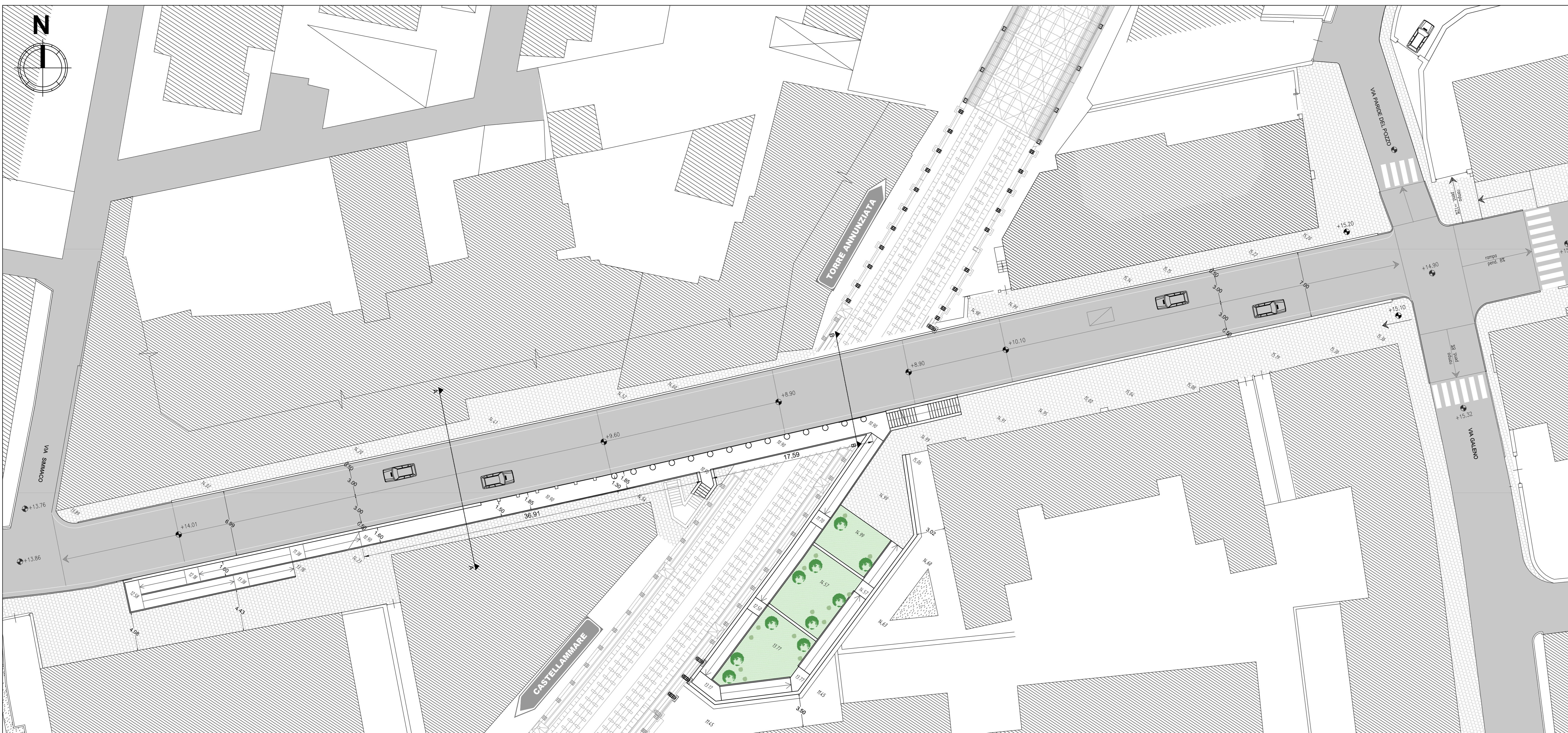
PLANIMETRIA GENERALE - Pianta quota strada Scala 1:200
