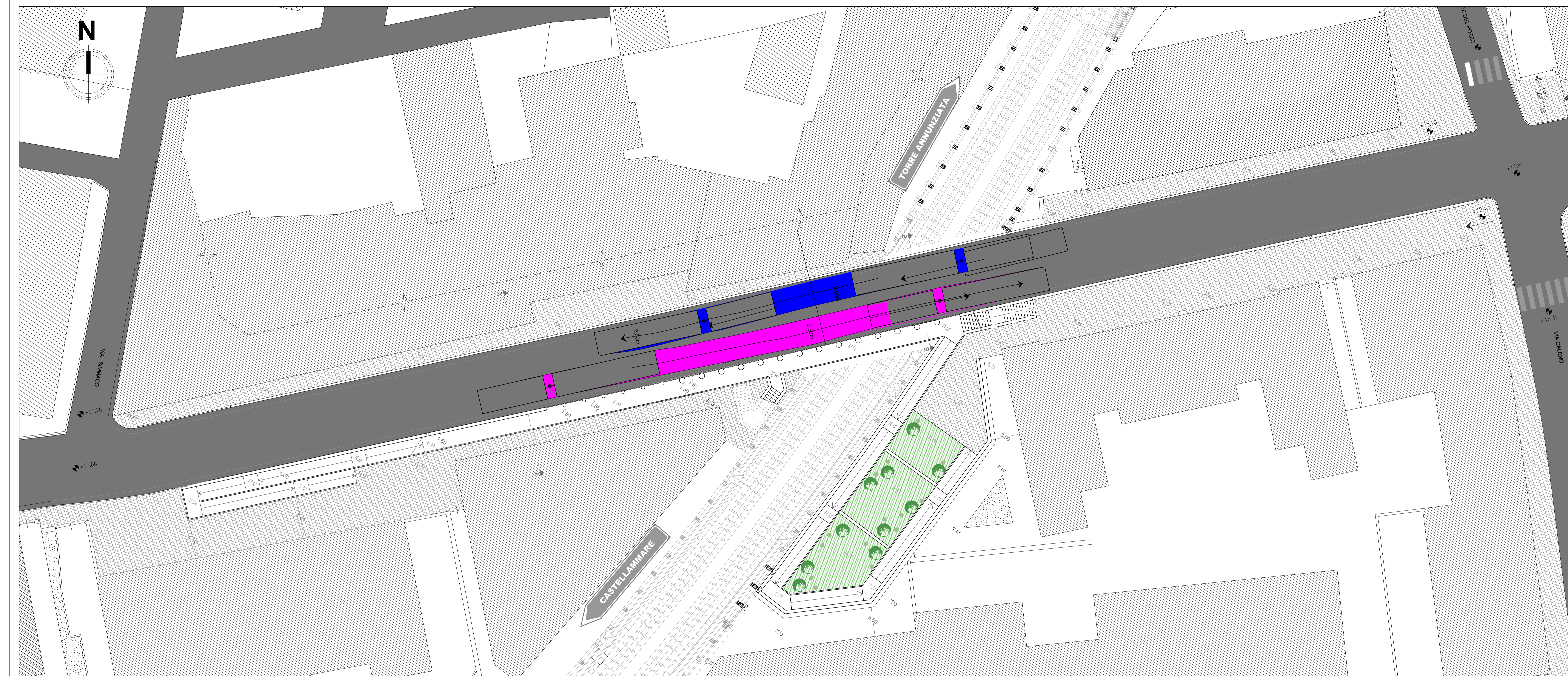
PLANIMETRIA GENERALE SOTTOPASSO - Pianta quota edifici - Ingombri planimetrici Scala 1:200
